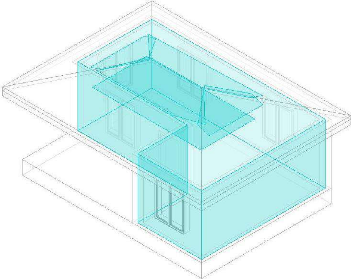
Görsel 3. Autodesk Revit programında oluşturulan enerji modeli
