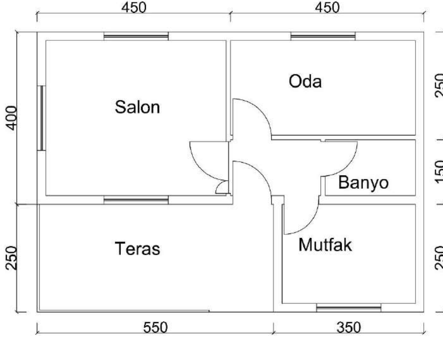
Görsel 1. Bağ evi modeli kat planı
