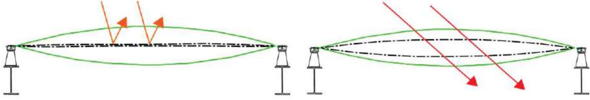
Görsel 2. Solda, basınç değeri azaltılarak ETFE folyoların birbirine yaklaştırılması ile yaz aylarında güneş erişimini sınırlayan dört katmanlı ETFE yastık diyagramı; sağda, basınç değeri artırılarak ETFE folyoların birbirinden uzaklaştırılması ile kış aylarında güneş erişimine izin veren dört katmanlı ETFE yastık diyagramı [7]
