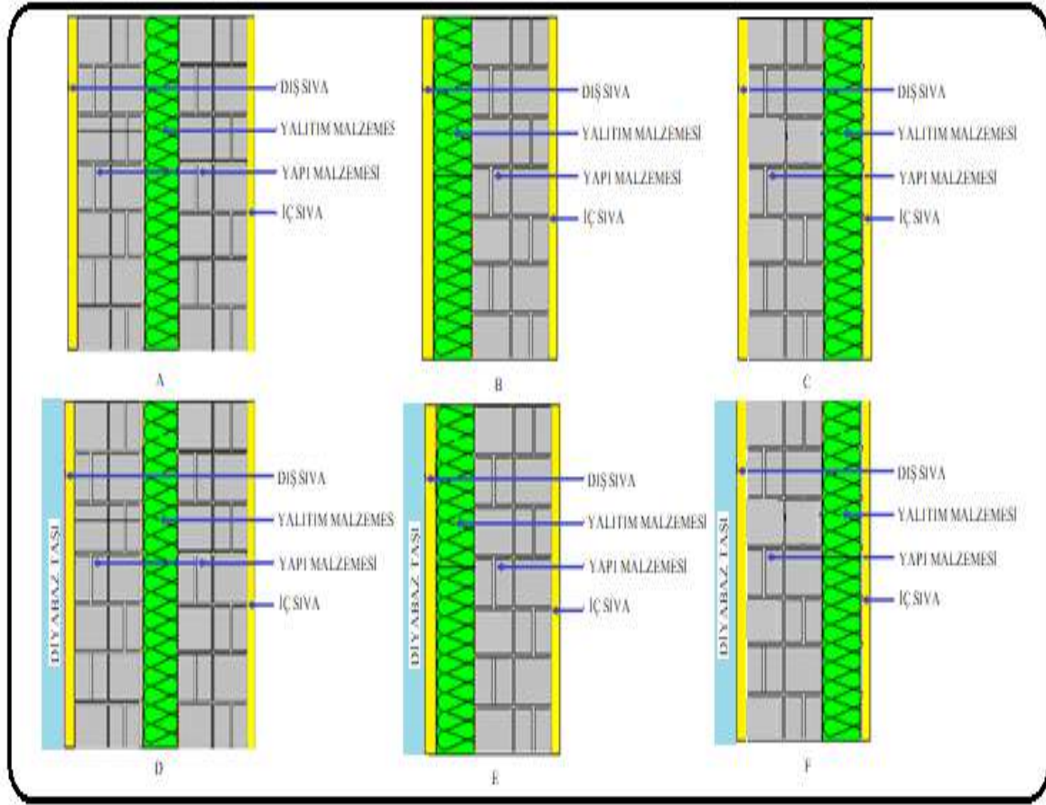
Görsel 4. Analizi Yapılan Duvar Yapıları
